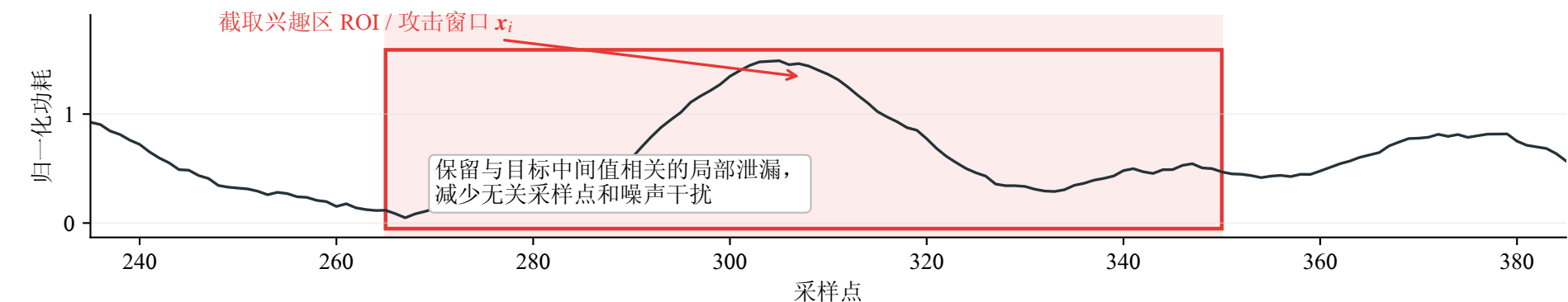
(b) 兴趣区截取：以第一轮 S 盒输出为目标截取局部攻击窗口
