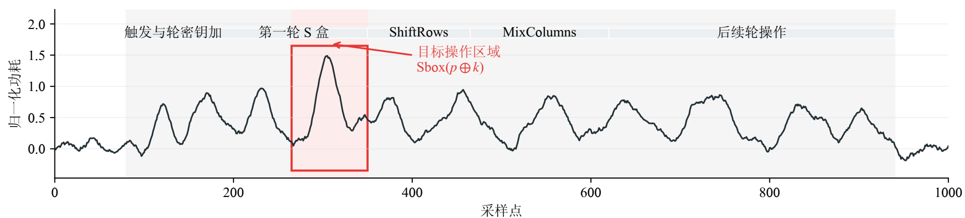
(a) 完整功耗曲线：从完整 AES 加密轨迹中定位目标 S 盒泄漏区域
