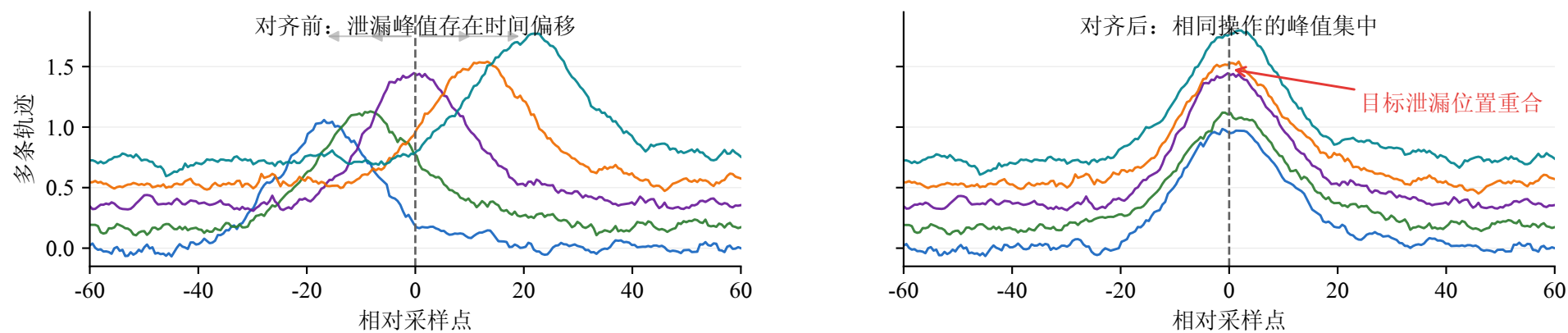
(c) 轨迹对齐前后对比：将同一密码操作对应的局部泄漏校准到相近采样位置
