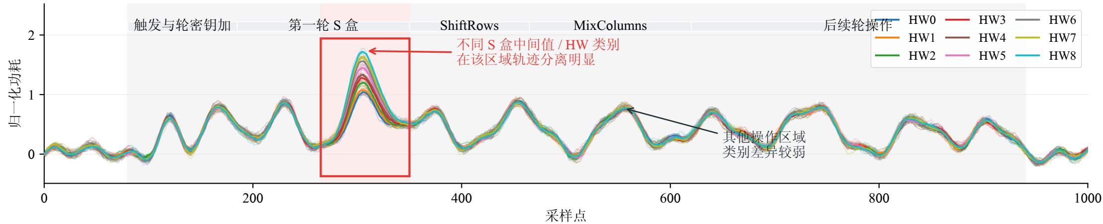
(a) 多条功耗轨迹：不同 S 盒中间值对应的轨迹在目标区域区分明显
