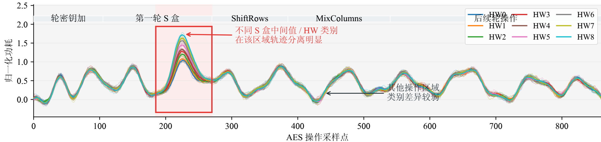
(a) AES 操作区间内的多条功耗轨迹：不同 S 盒中间值对应的轨迹在目标区域区分明显
