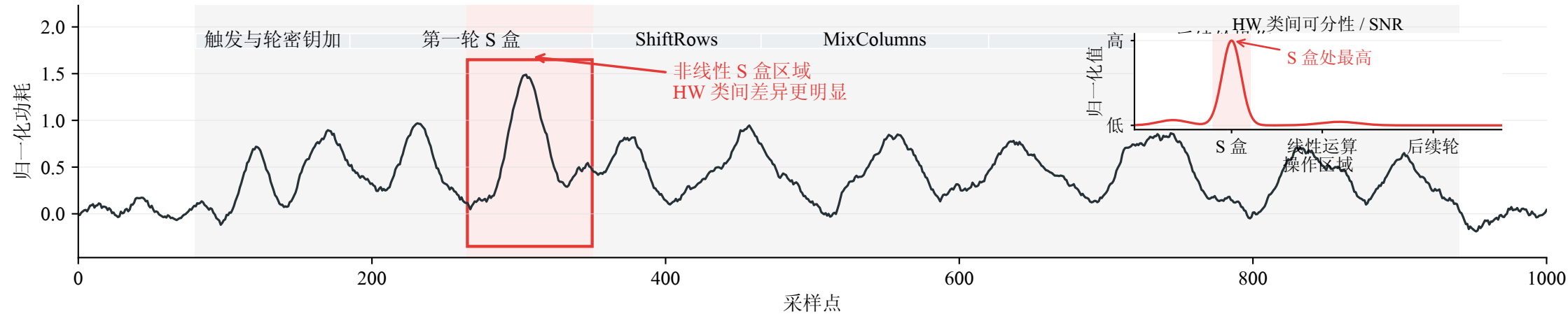
(a) 完整功耗曲线：第一轮 S 盒区域具有更明显的 HW 类间差异和更高的示意信噪比
