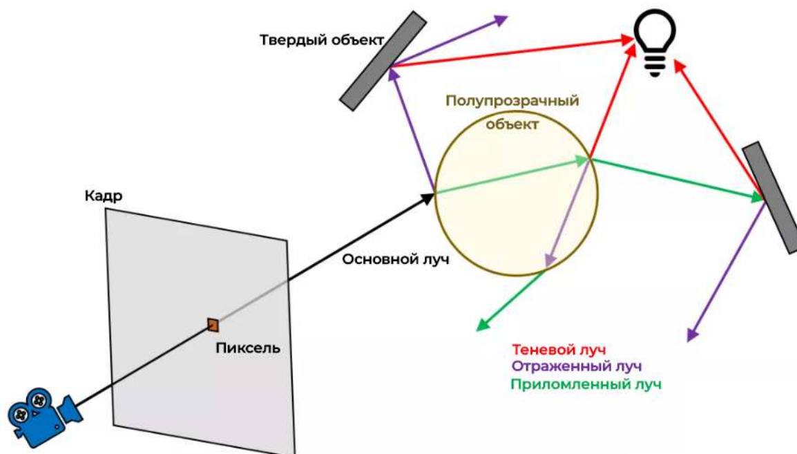
Рисунок 2 – Визуализация алгоритма трассировки путей
