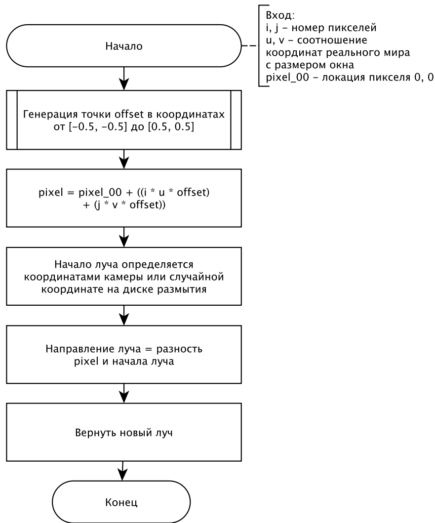
Рисунок 5 – Схема алгоритма генерации луча
