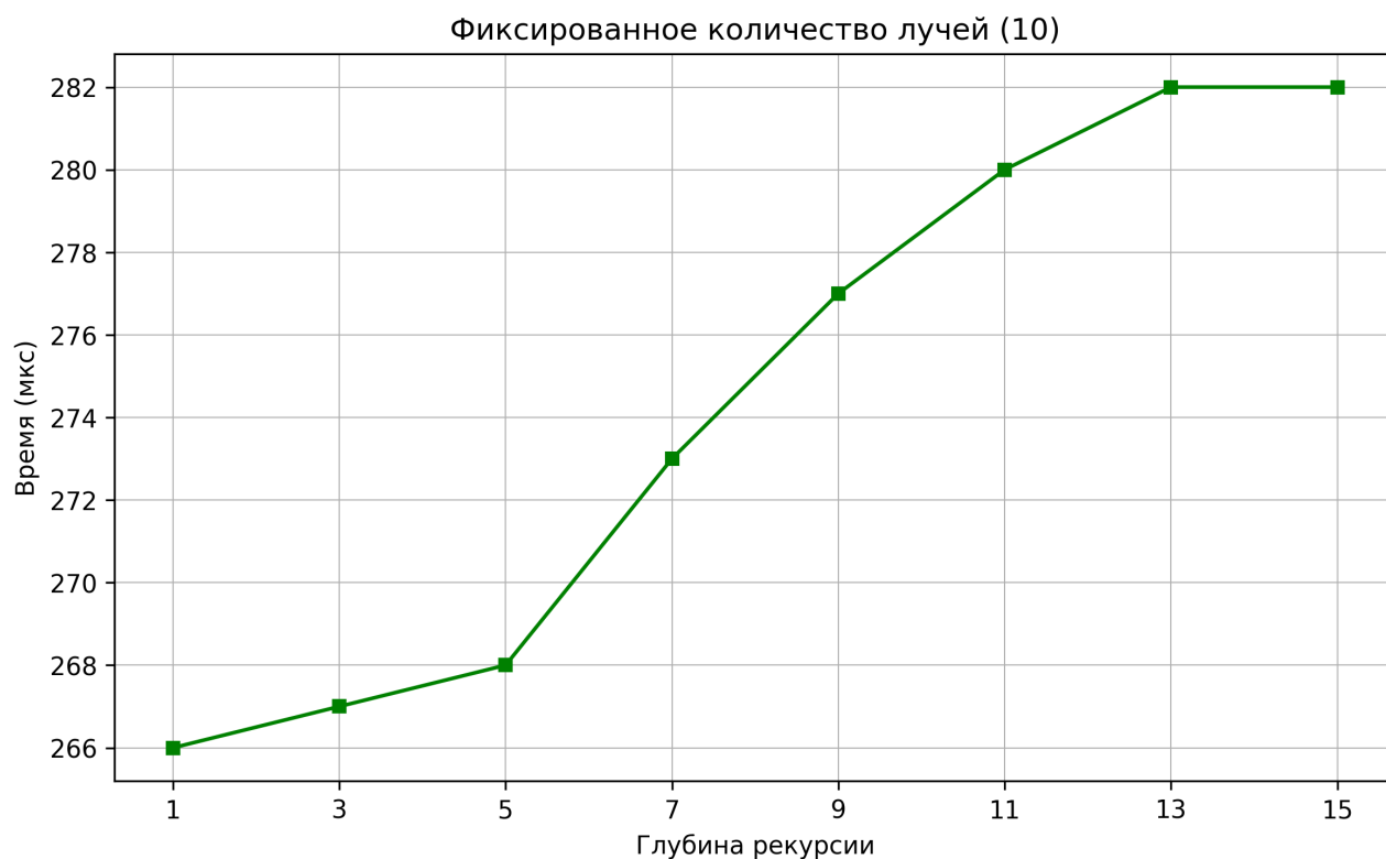
Рисунок 13 – график зависимости времени выполнения реализации алгоритма от максимального количества переотражений луча
