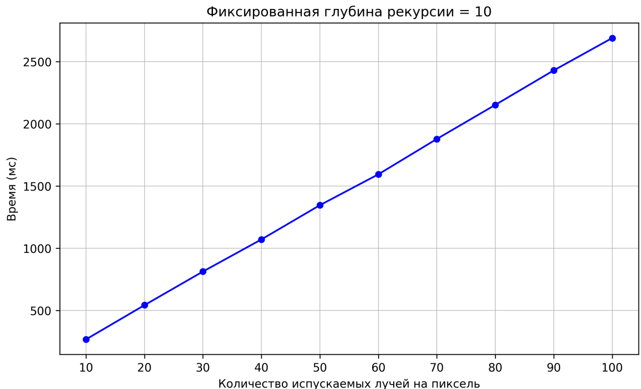
Рисунок 12 – график зависимости времени выполнения реализации алгоритма от количества лучей на пиксель
