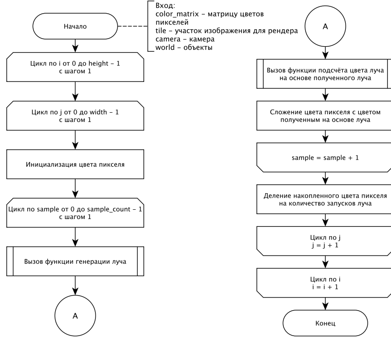
Рисунок 1 – Схема реализации алгоритма генерации части изображения
