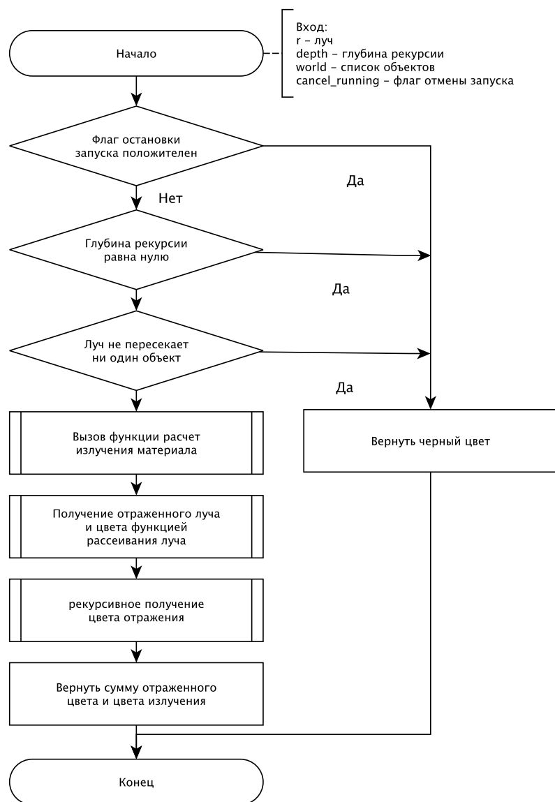
Рисунок 3 – Схема алгоритма рекурсивной трассировки пути
