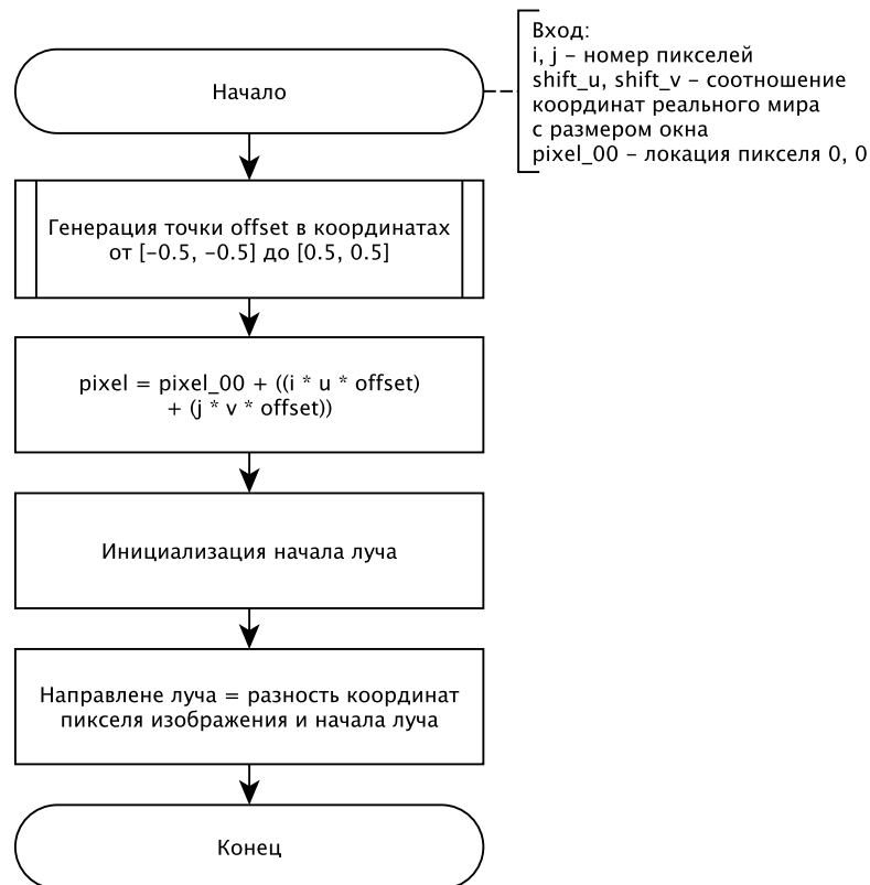
Рисунок 2 – Схема алгоритма генерации луча
