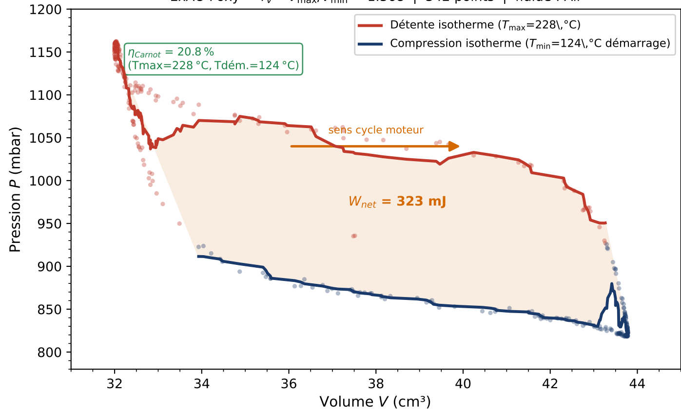
Diagramme P-V mesuré — Moteur Stirling Jeulin 204081 ExAO Foxy — r_v = V_{\max}/V_{\min} = 1.368 | 342 points | fluide : Air
