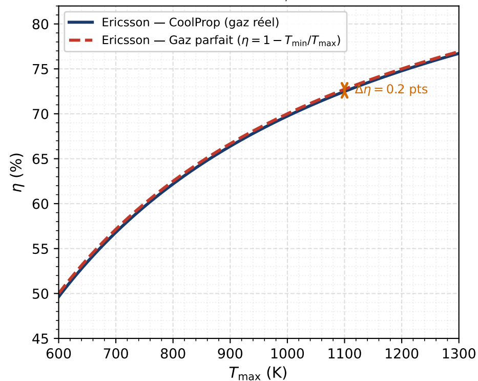
Ericsson : comparaison gaz parfait vs gaz réel (CoolProp) T_{\min} = 300 \text{ K} , r_p = 10 P_{\min} = 1 \text{ bar} , fluide : Air
