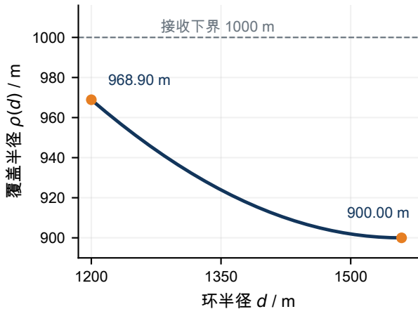
(a) 环增大，最坏覆盖距离缩短
