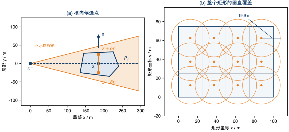
图 5: 中心横向测点与矩形光学覆盖示意
