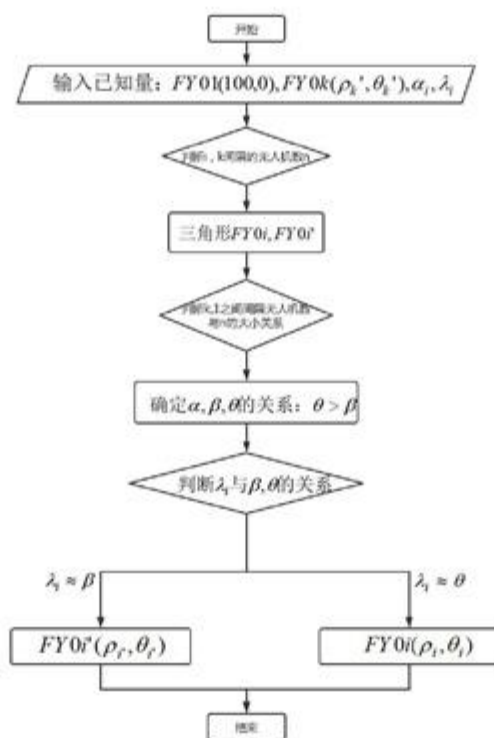
图 6-3 求解流程图
