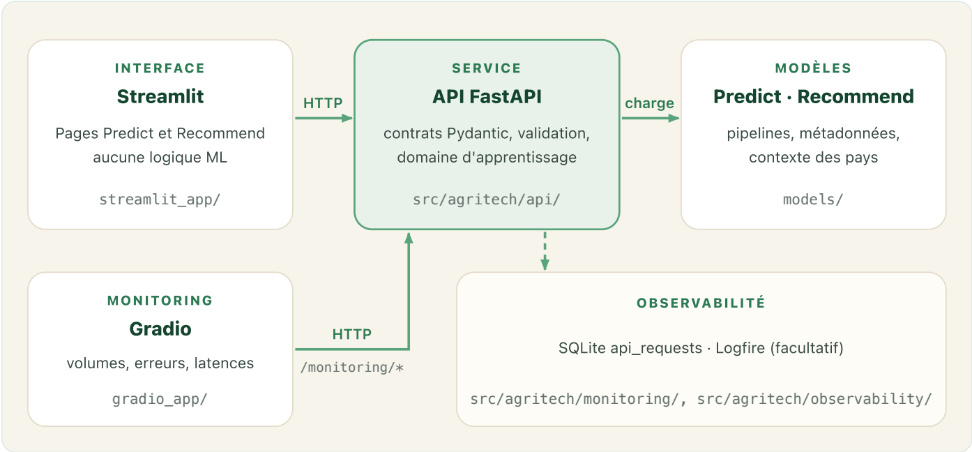
Architecture de l'application : l'interface Streamlit et le dashboard Gradio appellent l'API FastAPI, qui charge les modèles Predict et Recommend ; les appels /predict et /recommend sont archivés et tracés par la couche d'observabilité
