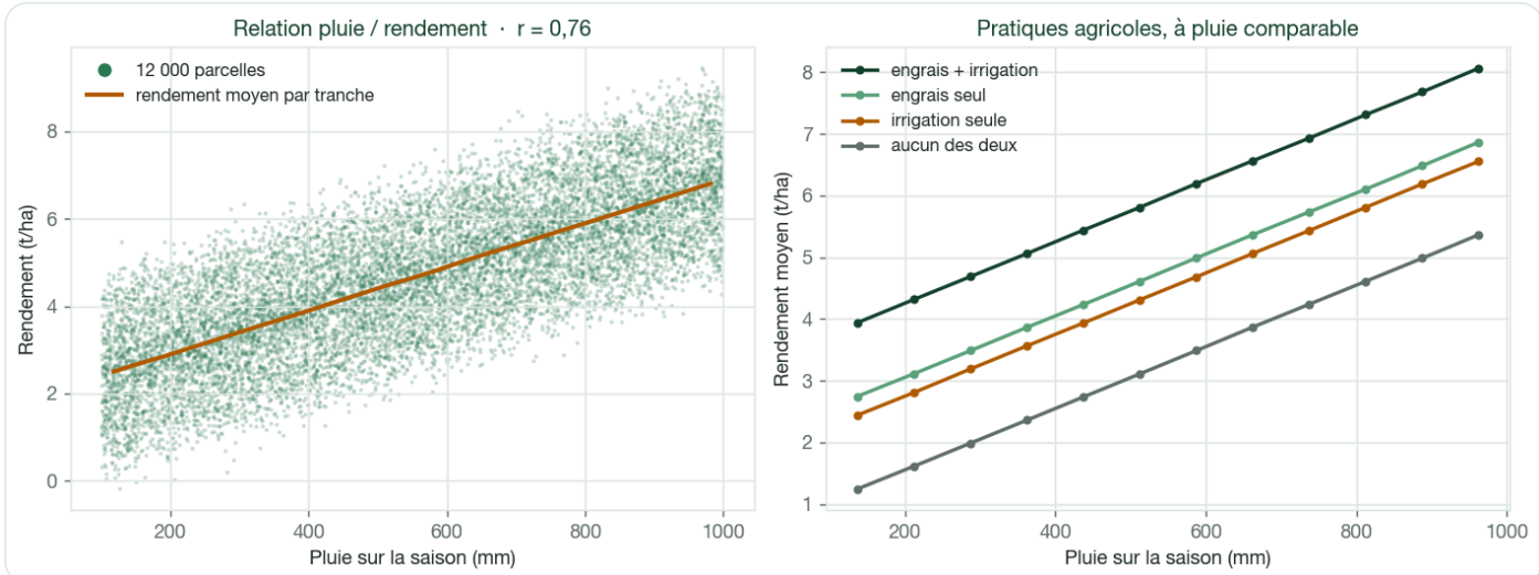
Relation pluie / rendement et rendement moyen selon les pratiques agricoles
