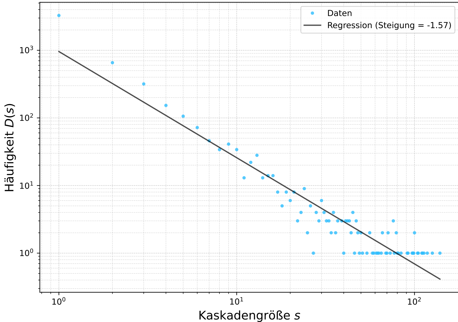
Häufigkeit einer Kaskade D(s) über dessen Größe s für L = 30
