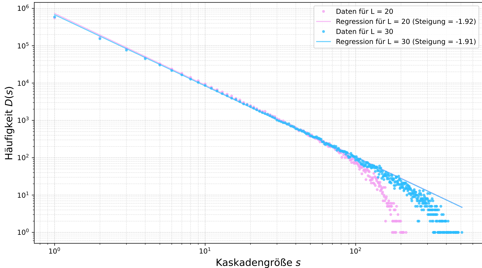
D(s) über s . Kumuliert über 21 runs für 50000 Durchläufe
