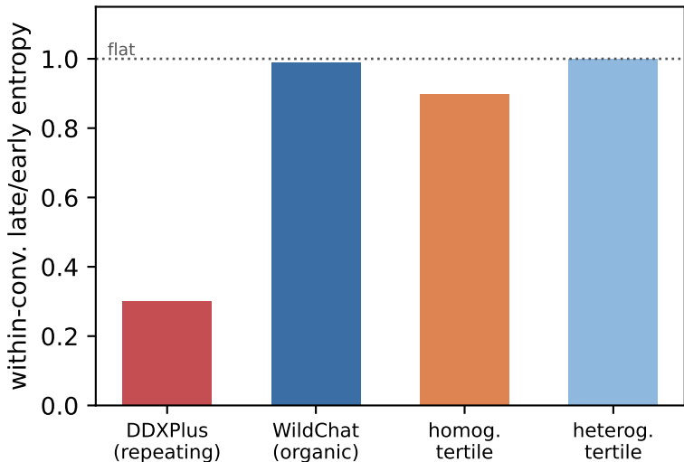
(d) Collapse needs a homogeneous task
