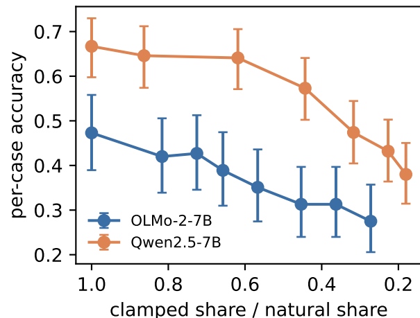
(d) The attention inversion
