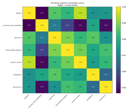
Claude labels
