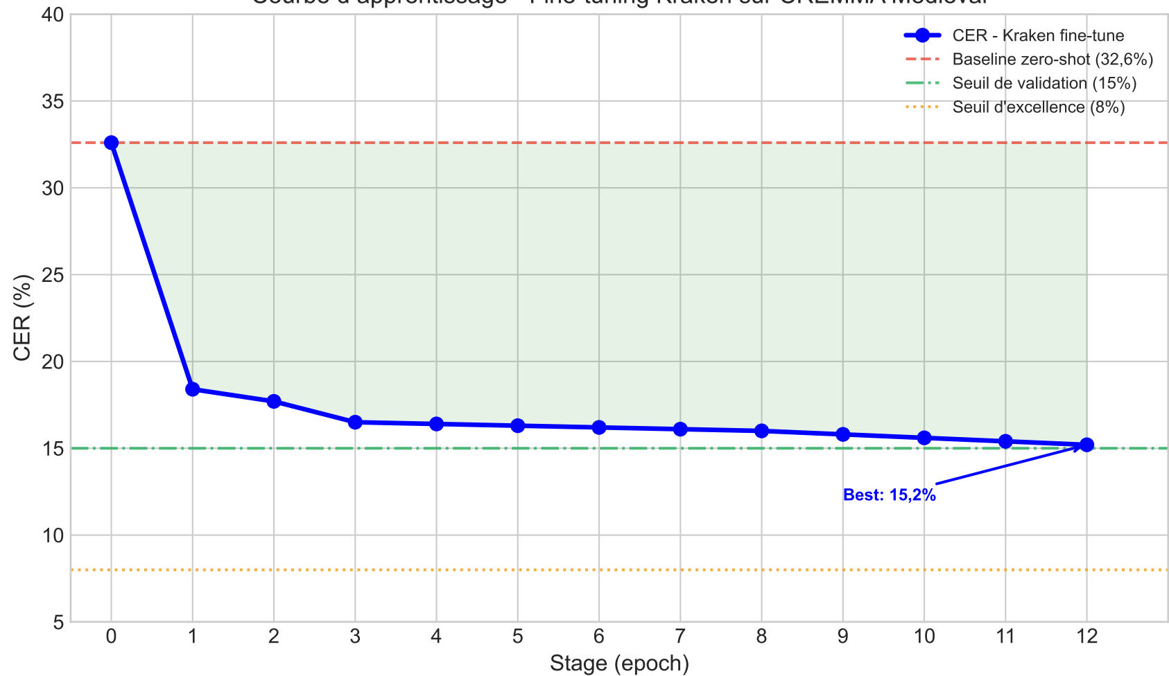
Courbe d apprentissage - Fine-tuning Kraken sur CREMMA Medieval
