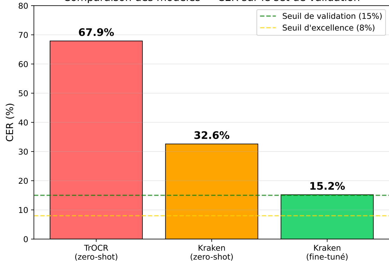
Comparaison des modèles — CER sur le set de validation
