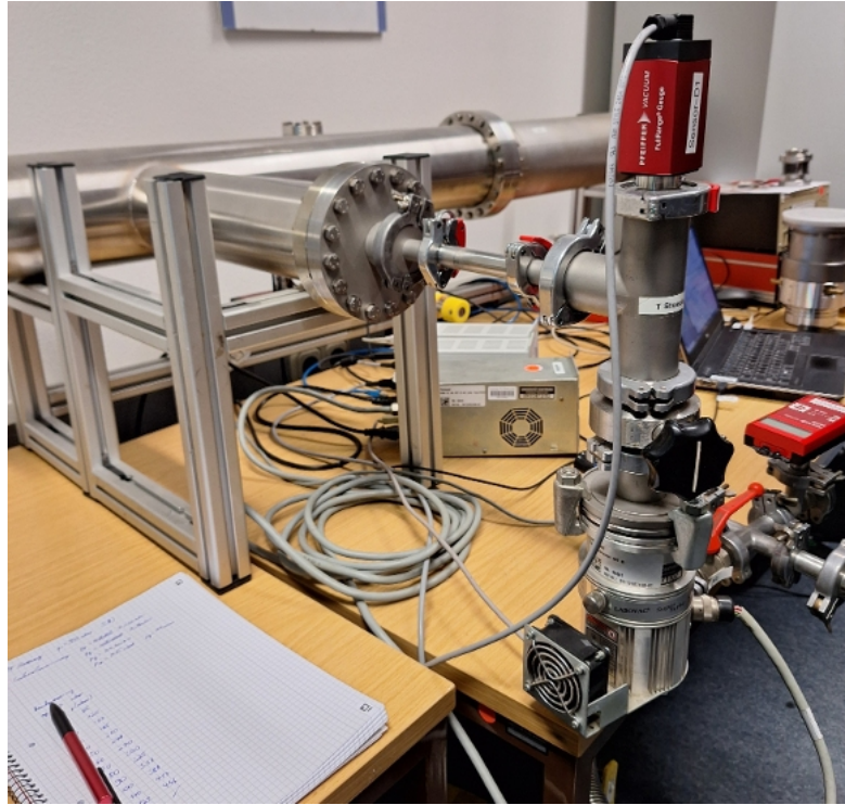
Abbildung 10: Eingebautes Testrohr zwischen TP und Rezipienten (Eigenaufnahme).
