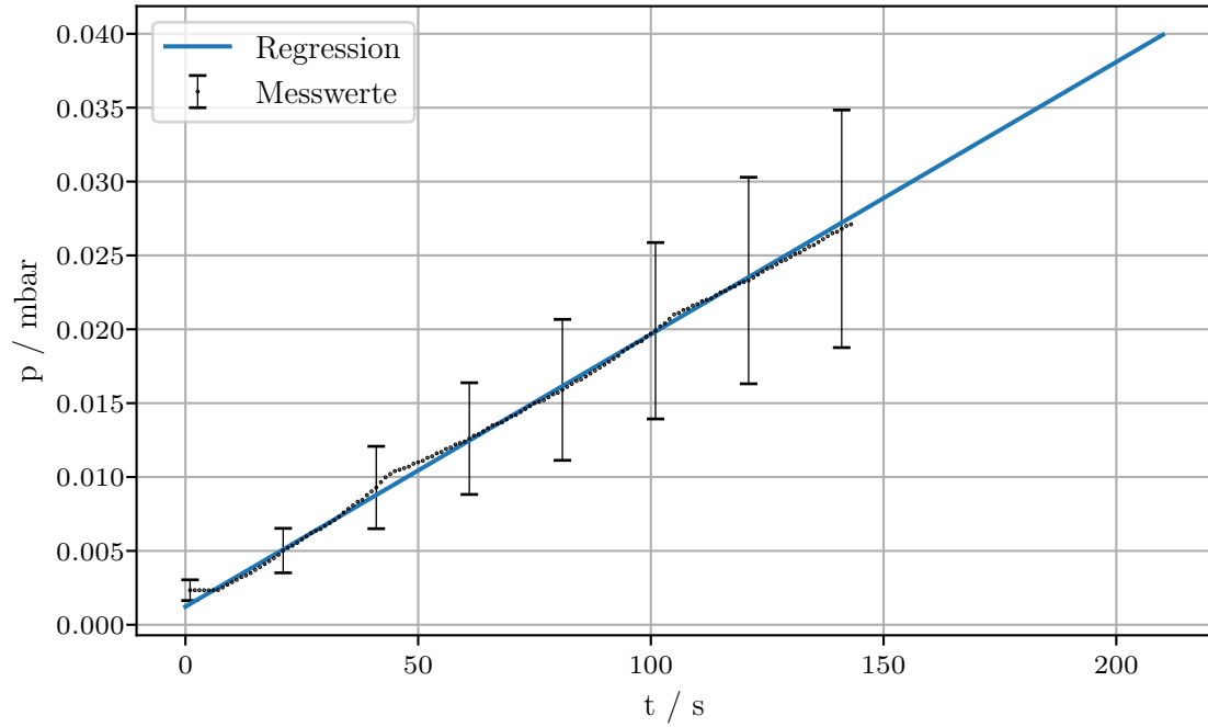
Abbildung 14: Ausgleichsrechnung zur bestimmung des Saugvermögens hinter der Engstelle
