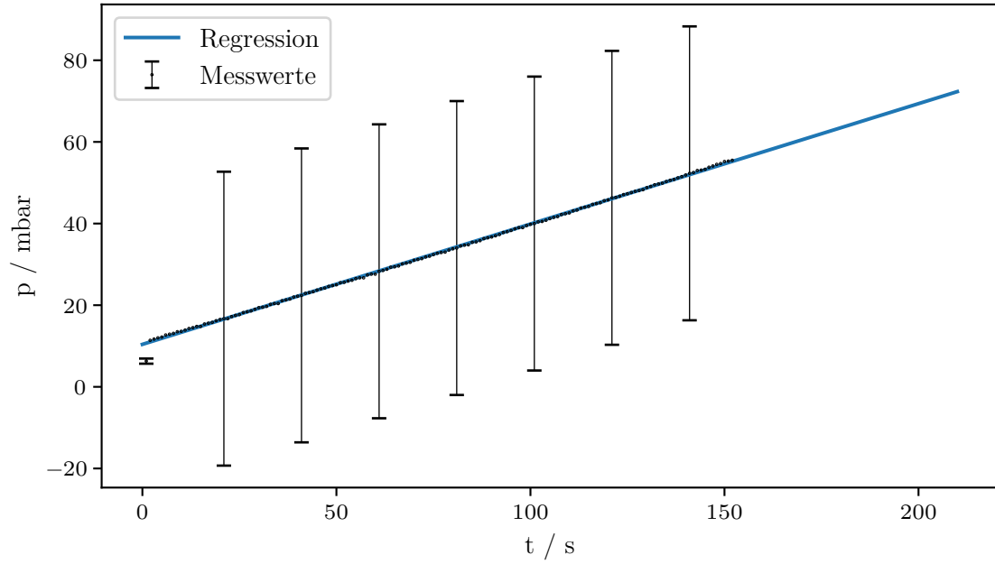
Leckratenmessung Drehschieberpumpe p_g = 10 \pm 4 mbar
