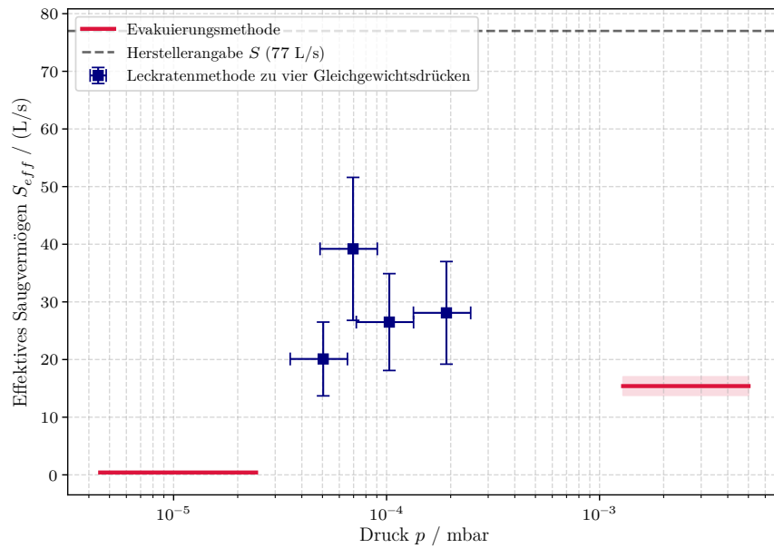
Abbildung 16: Saugvermögen der Turbomolekularpumpe in Abhängigkeit des Drucks.
