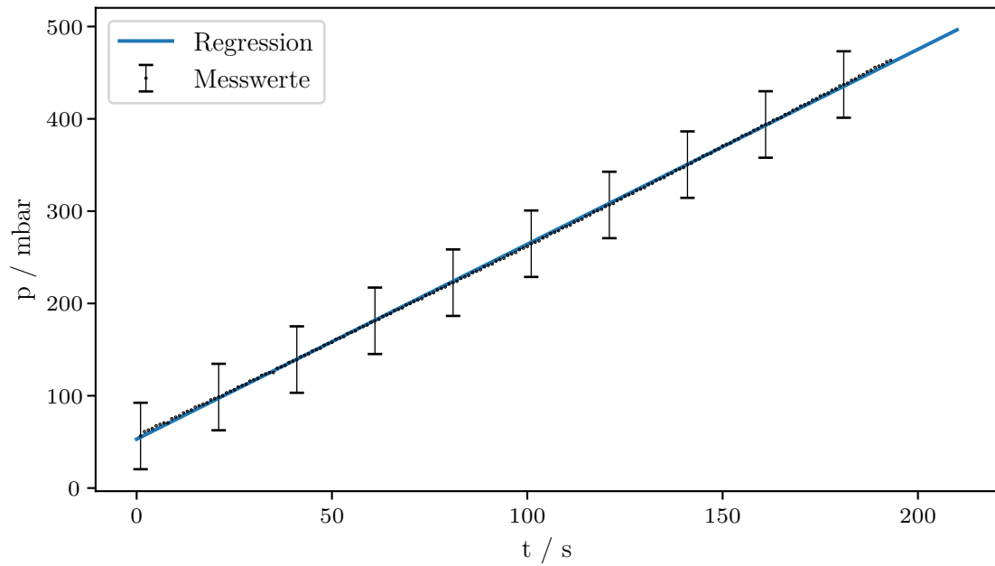
Leckratenmessung Drehschieberpumpe p_g = 50 \pm 4 mbar
