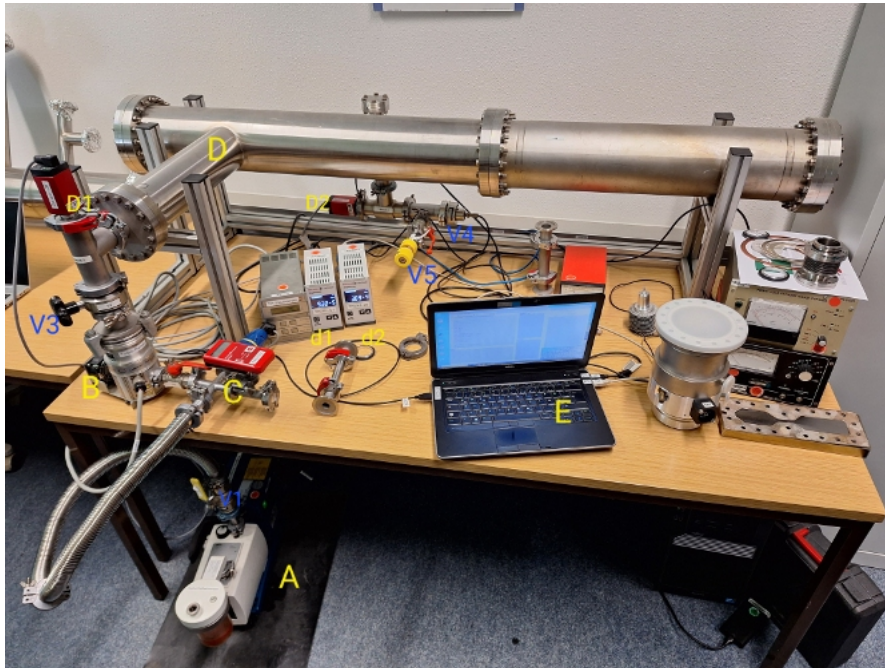
Abbildung 8: Aufbau der Apparatur (Eigenaufnahme).
