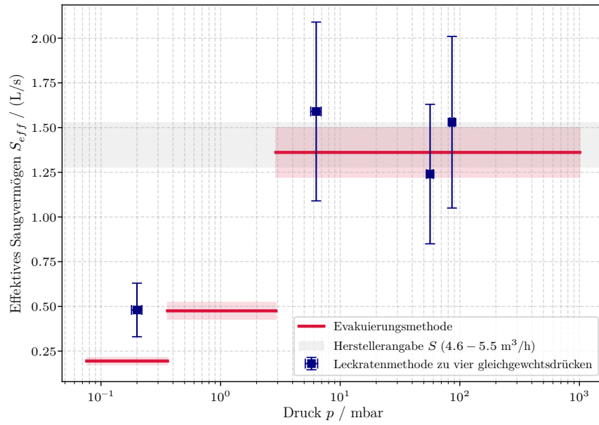
Abbildung 15: Saugvermögen der Drehschieberpumpe in Abhängigkeit des Drucks.
