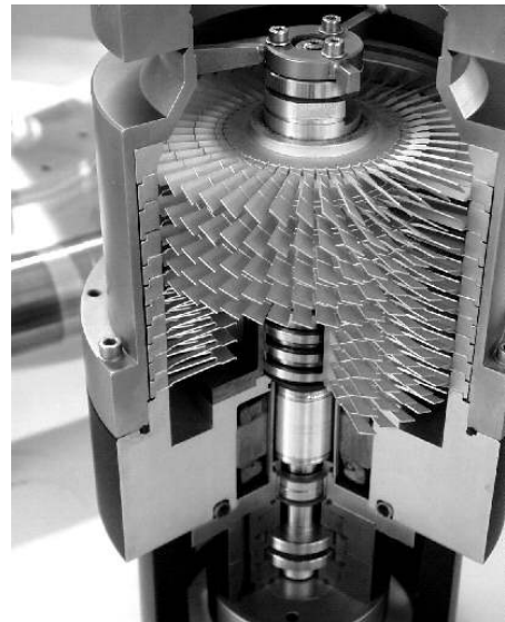
Abbildung 6: Innenleben der TMP. [5]
