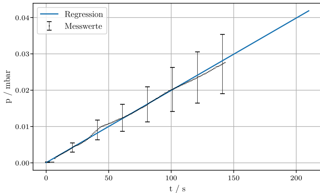
Abbildung 13: Ausgleichsrechnung zur bestimmung des Saugvermögens vor der Engstelle
