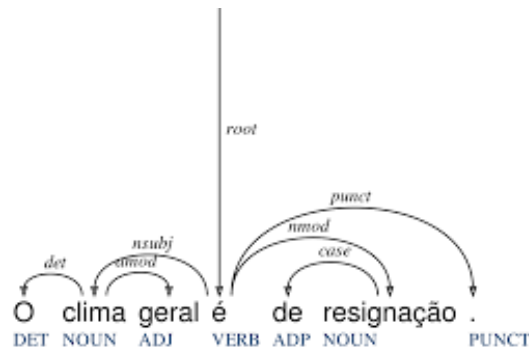
Figura 8 – Exemplo estrutural de uma árvore de análise por dependência sintática.
