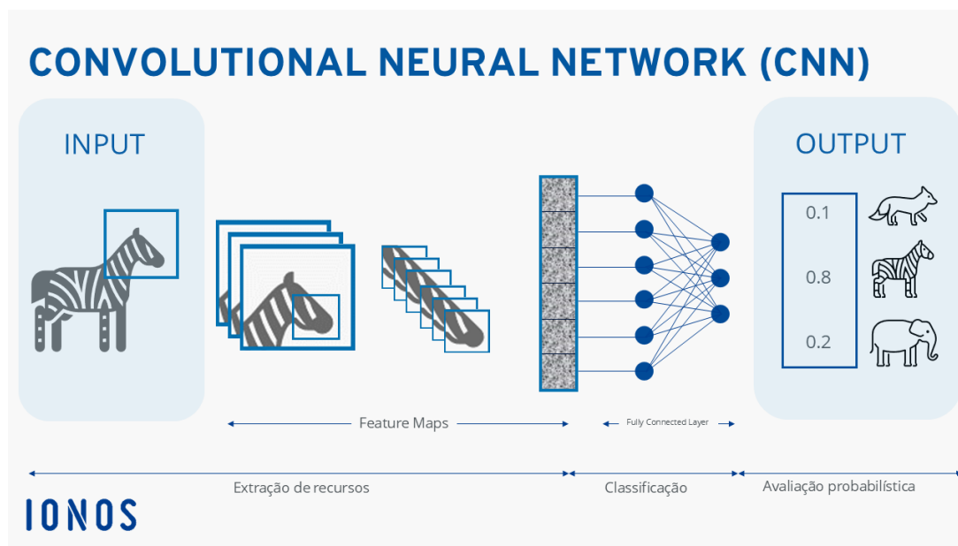
Figura 9 – Diagrama de blocos e fluxo de dados em uma Rede Neural Convolutiva.
