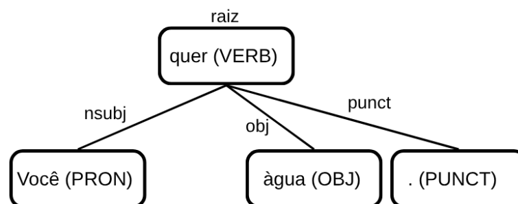
Figura 9 – Exemplo estrutural de uma árvore de análise por dependência sintática.
