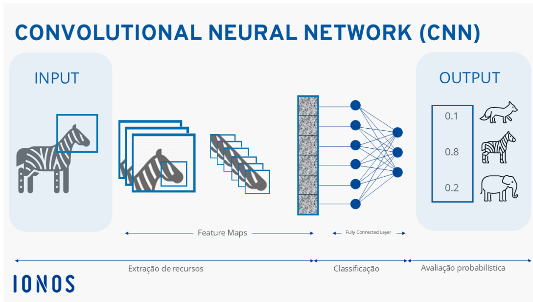
Figura 7 – Diagrama clássico de blocos e fluxo de dados em uma Rede Neural Convolutiva.
