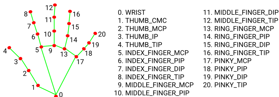
Figura 4 – Esquema dos 21 landmarks detectados pelo MediaPipe Hands .
