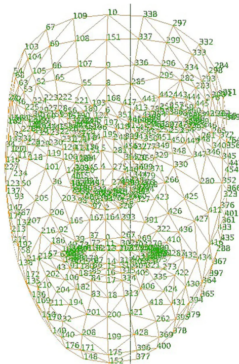
Figura 5 – Esquema dos 468 landmarks detectados pelo MediaPipe Face Mesh .
