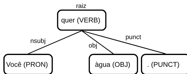
Figura 9 – Exemplo estrutural de uma árvore de análise por dependência sintática.
