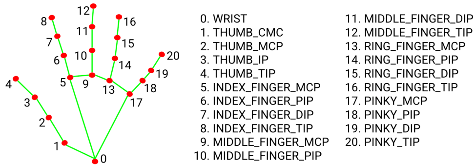
Figura 5 – Esquema dos 21 landmarks detectados pelo MediaPipe Hands .
