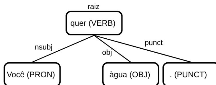
Figura 11 – Exemplo estrutural de uma árvore de análise por dependência sintática.
