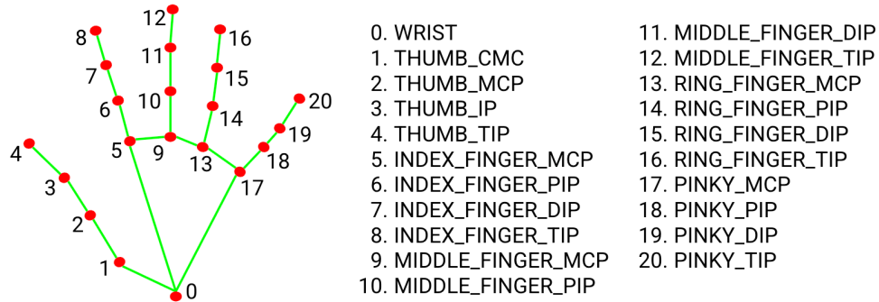
Figura 5 – Esquema dos 21 landmarks detectados pelo MediaPipe Hands .
