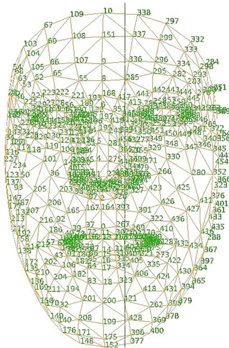
Figura 6 – Esquema dos 468 landmarks detectados pelo MediaPipe Face Mesh .
