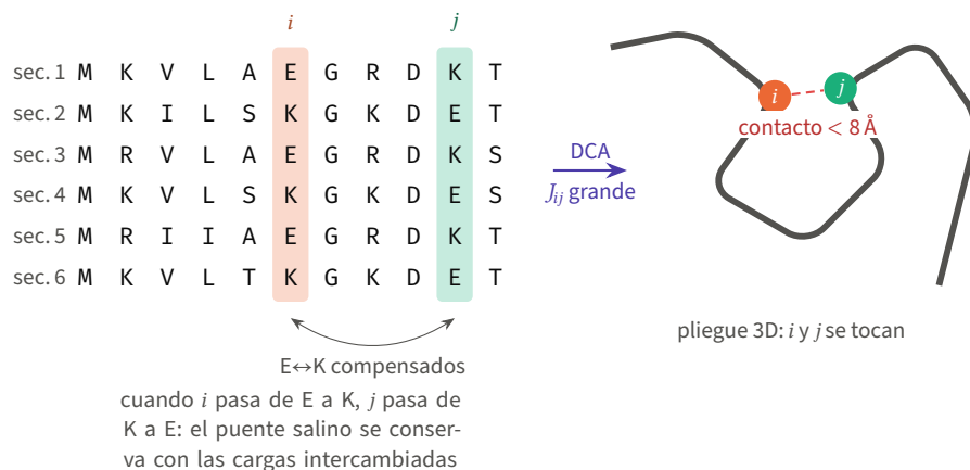
Figura 15.7. La señal de la coevolución. Izquierda: en un alineamiento de seis homólogos, las columnas i (naranja) y j (verde) cambian de forma coordinada: cuando i es glutamato (E), j es lisina (K), y viceversa, de modo que el puente salino entre ambos se conserva aunque los dos residuos cambien. Derecha: la explicación estructural más sencilla es que i y j están en contacto en el plegamiento. El análisis de acoplamiento directo (DCA) estima un acoplamiento J_{ij} por par, separando la covariación directa de la transmitida a través de terceros residuos.
