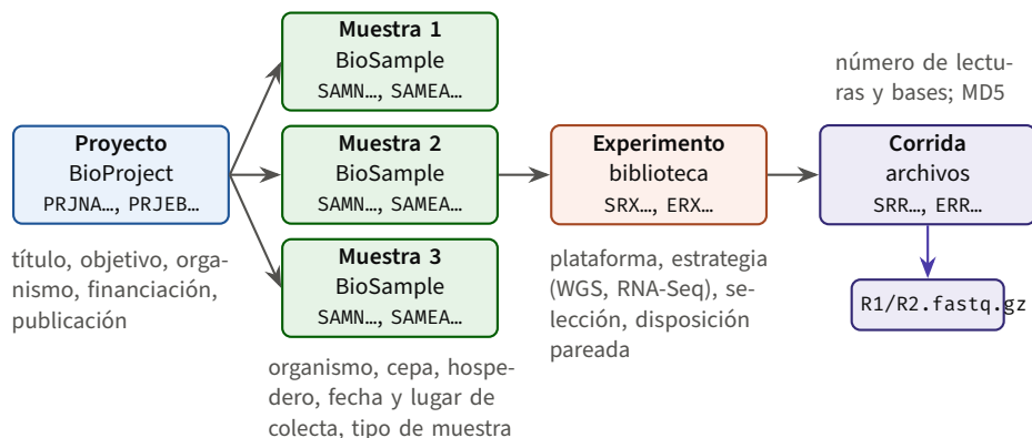
Figura 18.7. La jerarquía de objetos del SRA y el ENA, con los prefijos de sus accesiones (NCBI / EBI) y los metadatos que se describen en cada nivel. Un proyecto contiene muestras; cada muestra puede secuenciarse en varios experimentos (bibliotecas), y cada experimento en varias corridas. Las muestras llevan la información biológica que hará reutilizables los datos; los experimentos, la técnica. El artículo debe citar la accesión del proyecto, y el flujo debe descargar las lecturas por la accesión de cada corrida.
