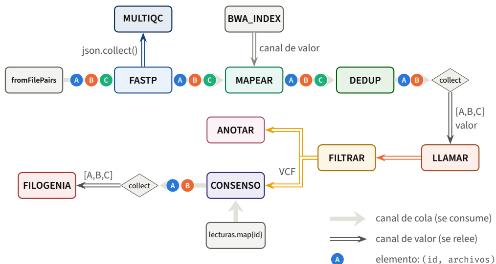
Figura 18.3. El mismo flujo de la figura 18.1 visto como flujo de datos en Nextflow. Los procesos (cajas) están aislados y solo se comunican por canales. Por los canales de cola (tubos grises) circulan elementos, uno por muestra, que cada proceso consume en cuanto llegan: la muestra A puede estar ya en DEDUP mientras C sigue en FASTP. El índice de BWA viaja por un canal de valor (doble línea) que MAPEAR relee para cada muestra, y el operador collect convierte la cola de BAM en un único valor, la lista completa, que dispara una sola vez el llamado conjunto. Lo mismo ocurre con el VCF filtrado, que CONSENSO relee para cada identificador de muestra, y con las secuencias consenso, que se reúnen antes de la filogenia.
