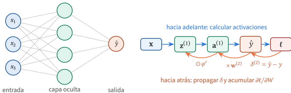
Figura 17.6. Izquierda: una red con tres entradas, una capa oculta de cuatro neuronas, a^{(1)} = \varphi(W^{(1)}x + b^{(1)}) , y una salida \hat{y} = \sigma(w^{(2)\top} a^{(1)} + b^{(2)}) (ecuación (17.16)); cada línea es un peso ajustable. Derecha: el mismo cálculo como grafo computacional. La pasada hacia adelante (azul) evalúa las activaciones y la pérdida \ell ; la pasada hacia atrás (naranja) propaga la “señal de error” \delta desde la pérdida hasta la entrada, multiplicando en cada paso por la derivada local (teorema 17.2). El coste de la pasada hacia atrás es del mismo orden que el de la pasada hacia adelante.
