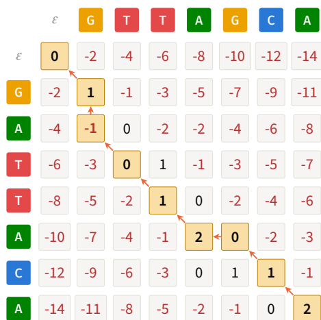
Figura 3.5. Matriz de programación dinámica para x = \text{GATTACA} (filas) e y = \text{GTTAGCA} (columnas), con s = +1 para coincidencias, -1 para sustituciones y d = 2 . Las celdas resaltadas y las flechas naranjas marcan el traceback desde la esquina inferior derecha. Los valores negativos aparecen en rojo.
