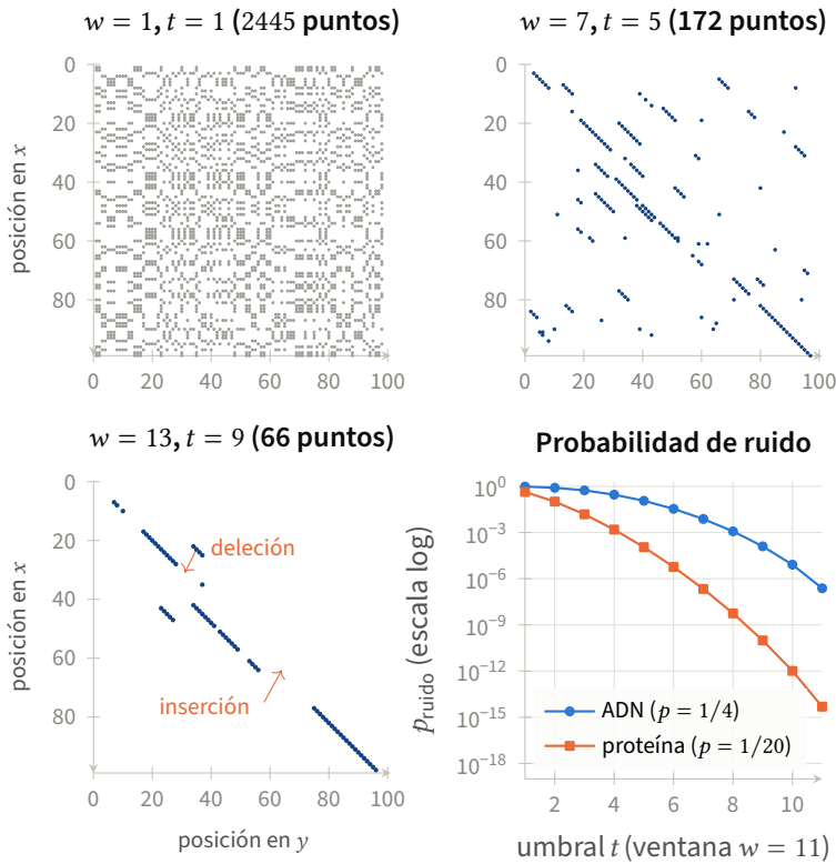
Figura 3.1. El mismo par de secuencias de ADN simuladas (100 pb; y es una copia de x con 15 % de sustituciones, una deleción de 8 pb y una inserción de 6 pb) visto con tres filtros distintos. Con w = t = 1 (arriba a la izquierda) una cuarta parte de las celdas tiene un punto y la diagonal verdadera se ahoga en el ruido. Con w = 7, t = 5 la diagonal emerge, y con w = 13, t = 9 el ruido casi desaparece y se leen los dos indels como saltos laterales de la diagonal (flechas). Abajo a la derecha, la ecuación (3.2) para w = 11 : con 20 letras el ruido cae mucho más rápido que con 4, por eso los dot plots de proteínas toleran ventanas más cortas. Datos de figuras/cap03/generar.py .
