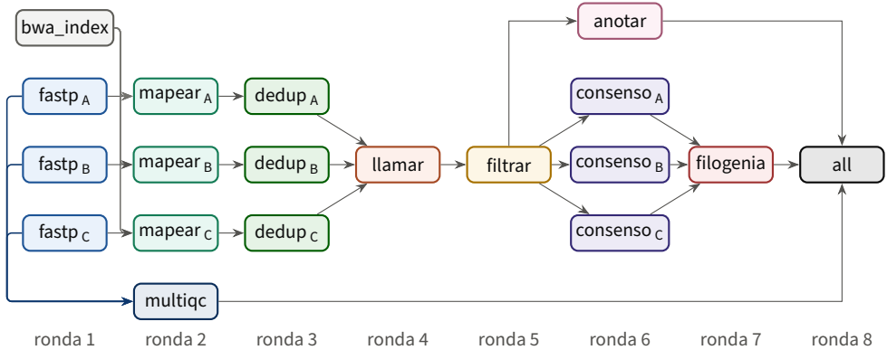
Figura 18.1. Grafo de trabajos del flujo de ejemplo con tres muestras (A, B, C): de lecturas crudas a variantes anotadas, secuencias consenso, un árbol filogenético y un informe de calidad. Cada color es una regla del Snakefile de la sección 18.1.5; los subíndices son los valores del comodín m . Las columnas son las rondas del algoritmo de Kahn: todos los trabajos de una ronda son independientes entre sí y pueden ejecutarse a la vez (anchos 4, 4, 3, 1, 1, 4, 1, 1). Observe los dos cuellos de botella de anchura 1, llamar y filtrar : el llamado conjunto necesita todas las muestras, y por ahí pasa todo el flujo. El índice de BWA (gris) se construye una sola vez y alimenta los tres mapeos; los tres informes de fastp confluyen en multiqc (azul oscuro, abajo). Grafo calculado con figuras/cap18/generar.py .
