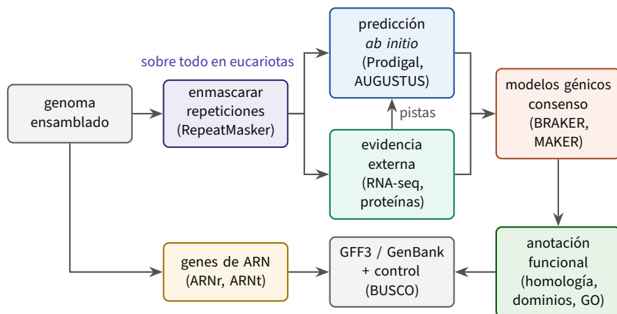
Figura 8.11. Flujo típico de anotación. Las repeticiones se enmascaran primero para que sus marcos de lectura (transposasas, transcriptasas inversas) no se confundan con genes del huésped. La predicción ab initio usa solo la secuencia y un modelo estadístico entrenado para la especie; la evidencia externa (transcritos de RNA-seq alineados, proteínas de especies cercanas) se incorpora como “pistas” que el predictor debe respetar o como modelos independientes que después se combinan. Los genes de ARN estructurales se buscan con modelos propios. Por último, a cada gen se le asigna una función por homología y el conjunto se valida, por ejemplo, con BUSCO en modo proteína. En procariotas, herramientas como Prokka y Bakta automatizan todo el flujo.
