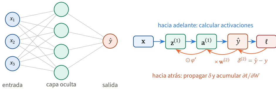
Figura 17.6. Izquierda: una red con tres entradas, una capa oculta de cuatro neuronas, a^{(1)} = \varphi(W^{(1)}x + b^{(1)}) , y una salida \hat{y} = \sigma(w^{(2)\top}a^{(1)} + b^{(2)}) (ecuación (17.16)); cada línea es un peso ajustable. Derecha: el mismo cálculo como grafo computacional. La pasada hacia adelante (azul) evalúa las activaciones y la pérdida \ell ; la pasada hacia atrás (naranja) propaga la “señal de error” \delta desde la pérdida hasta la entrada, multiplicando en cada paso por la derivada local (teorema 17.2). El coste de la pasada hacia atrás es del mismo orden que el de la pasada hacia adelante.
