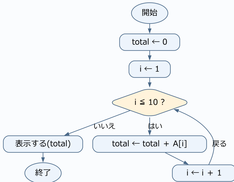
演習6-Aのフローチャート
