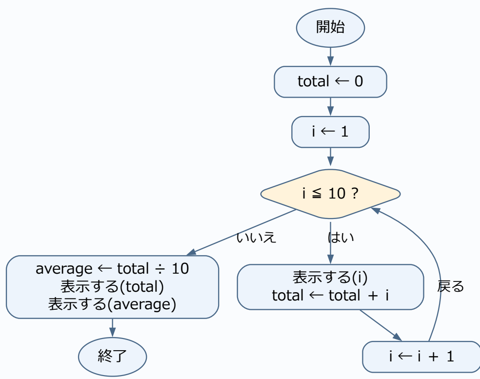
演習5-Aのフローチャート
