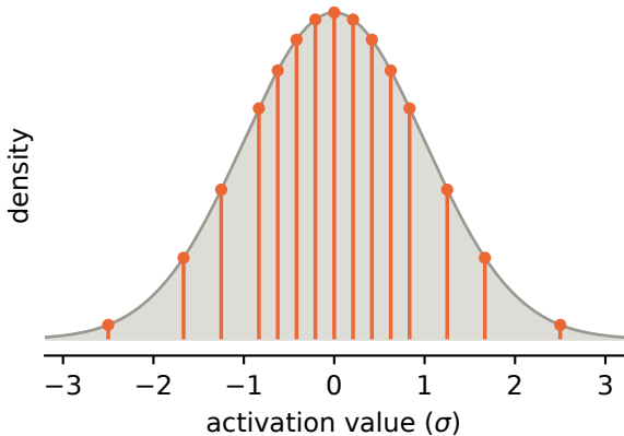
(a) FP4 (E2M1) · 19.2 dB SNR
