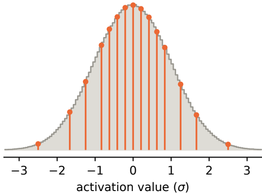
(a) FP4 (E2M1) · 19.2 dB SNR
