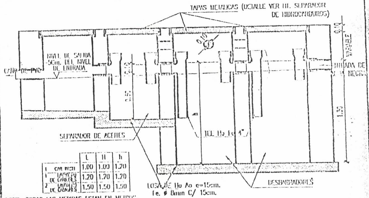
CORTE A-B
