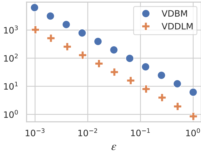
L1 error
