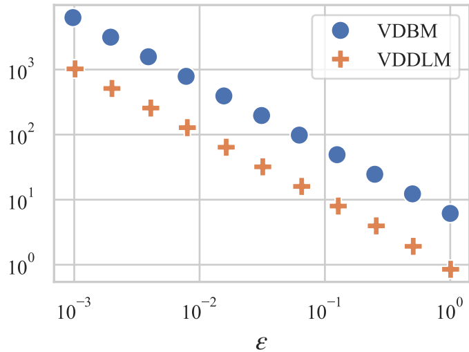
L1 error
