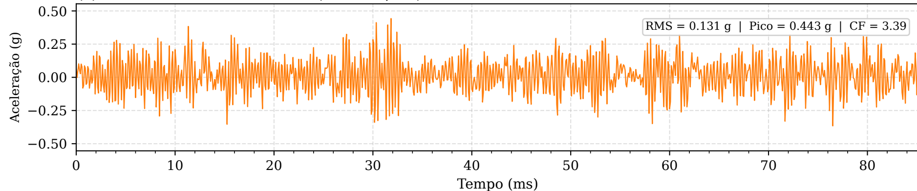
(d) Falha no Elemento Rolante (Ball — 0,07")
