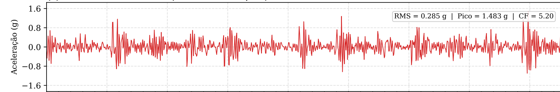
(b) Falha na Pista Interna (Inner Race — 0,07")
