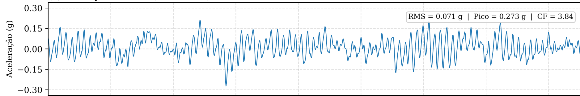
(a) Condição Normal (Sem Falha)
