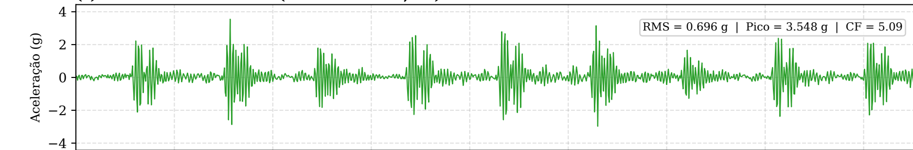
(c) Falha na Pista Externa (Outer Race — 0,07")
