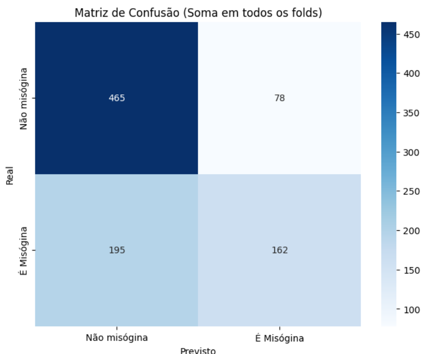
Figura 5.4: Matriz de Confusão do modelo: Soma dos resultados em todos os folds
