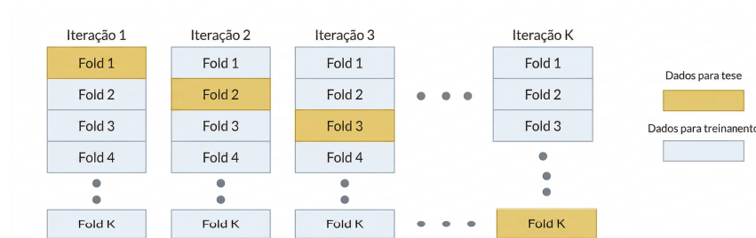
Figura 2.1: Ilustração dos conjuntos de dados sendo utilizados para as etapas de treino e teste gerados no procedimento de validação cruzada K -Fold
