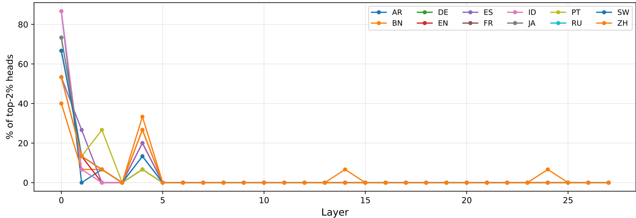
Qwen-2.5-7B (SFT)
