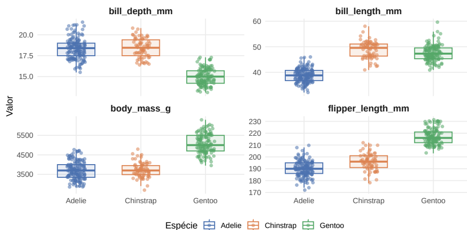
Figura 2: Distribuição das Variáveis Numéricas por Espécie
