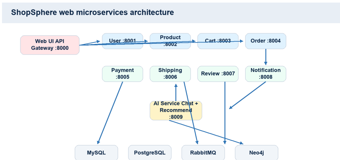
Hình 4.5. Sơ đồ kiến trúc hệ thống khi triển khai local
