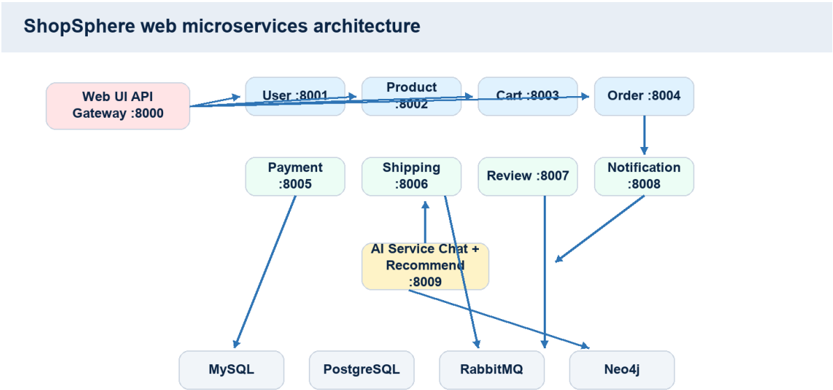
Hình 4.4. Component Diagram toàn hệ thống ShopSphere
