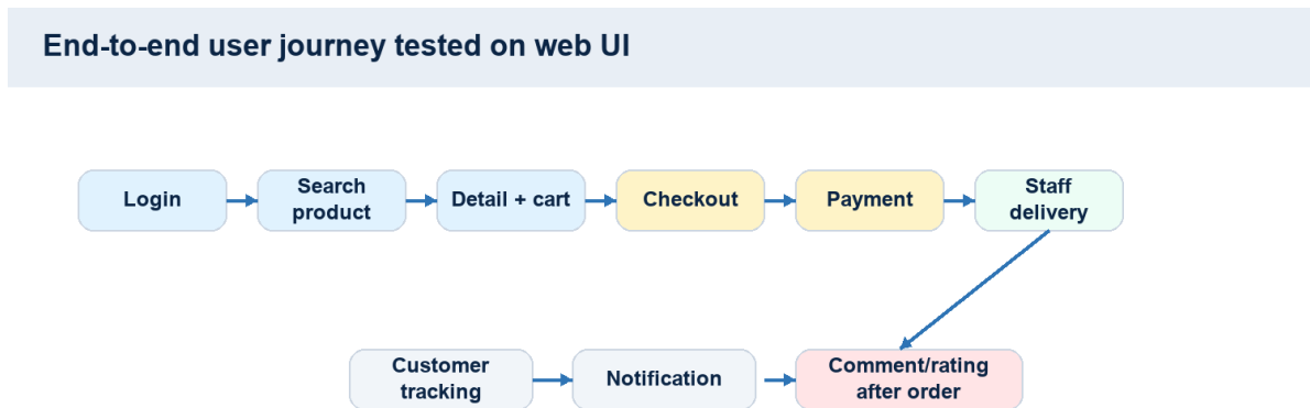
Hình 4.7. Sơ đồ hành trình mua hàng hoàn chỉnh trên ShopSphere
