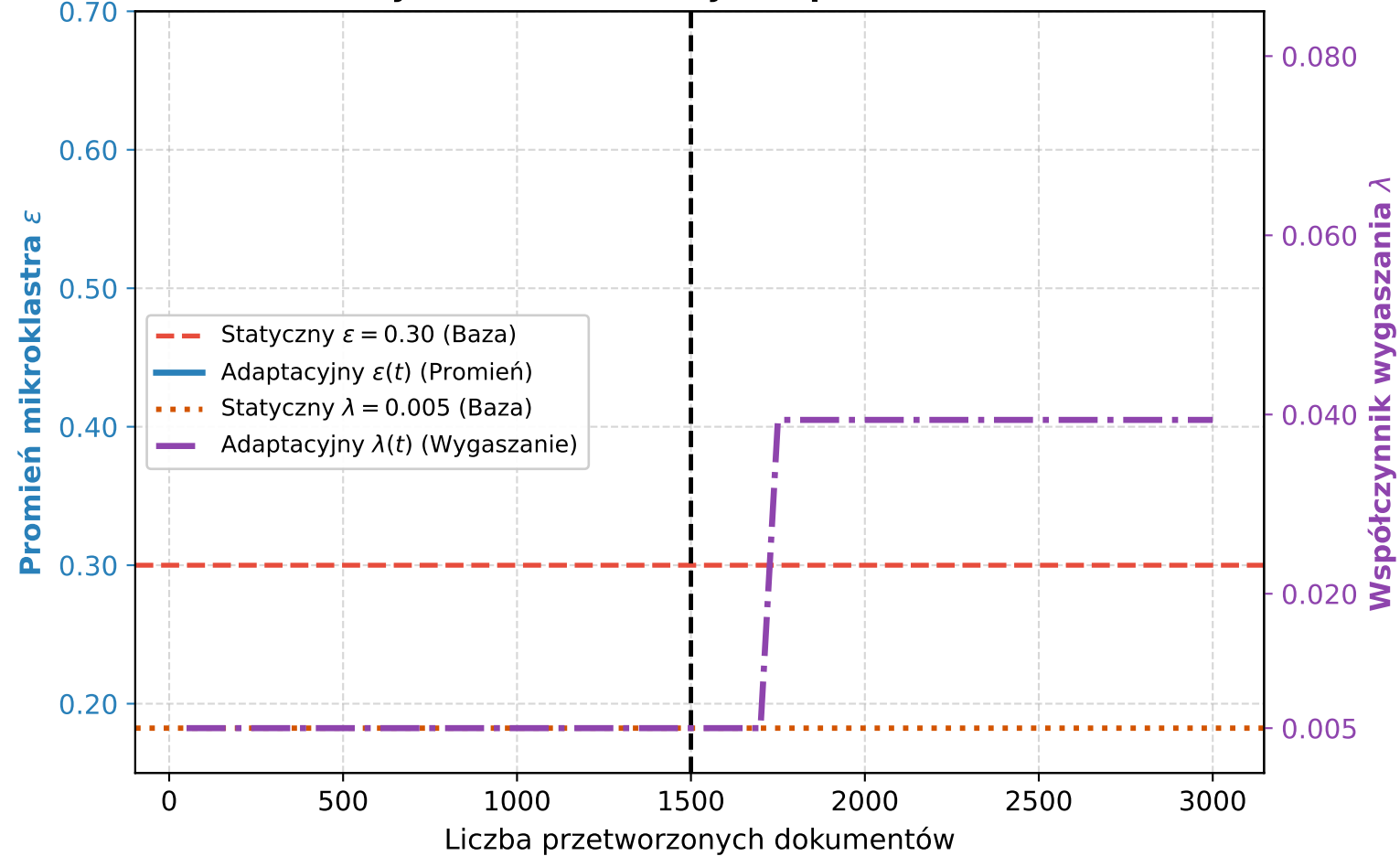
(c) Trajektoria samostrojzenia parametrów ( \epsilon, \lambda )
