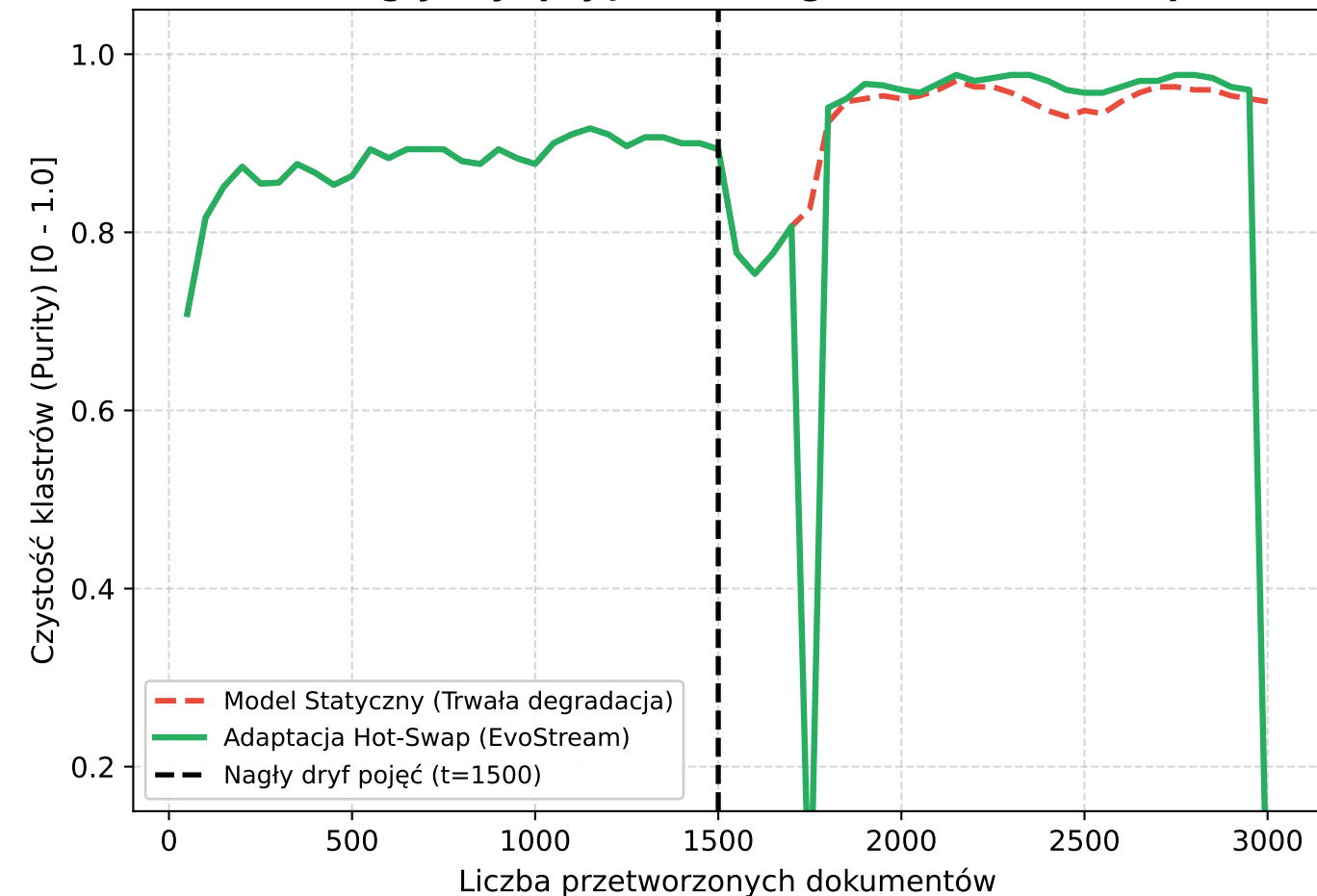
(b) Nagły dryf pojęć: Przewaga modelu Hot-Swap
