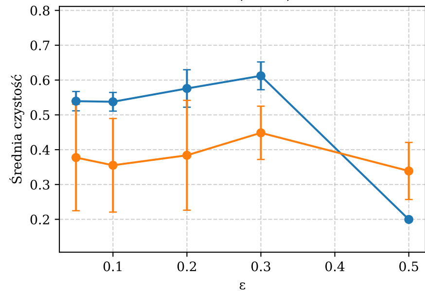
IPCA (d=32)
