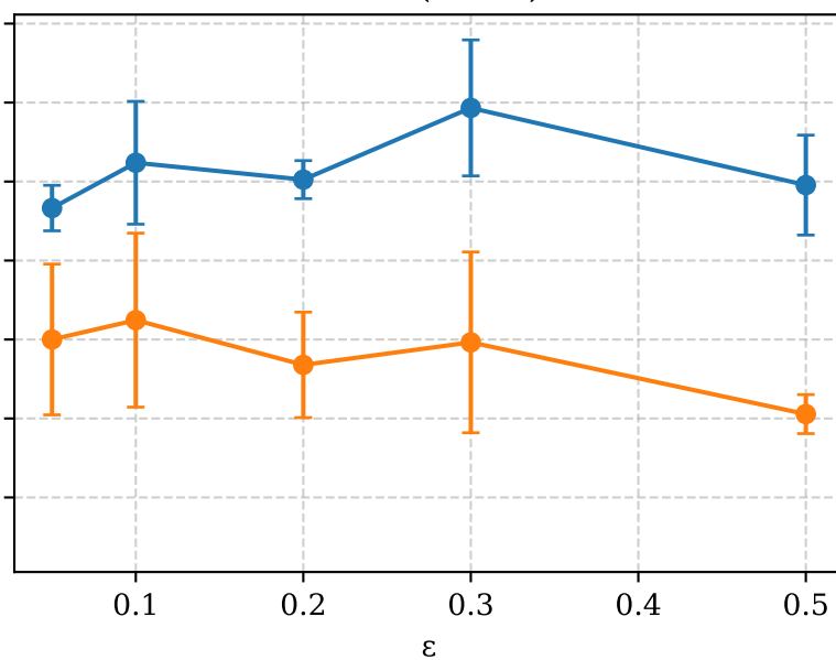
IPCA (d=16)
