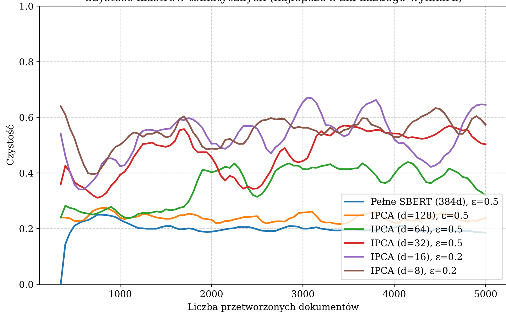
Czystość klastrow tematycznych (najlepsze \varepsilon dla każdego wymiaru)
