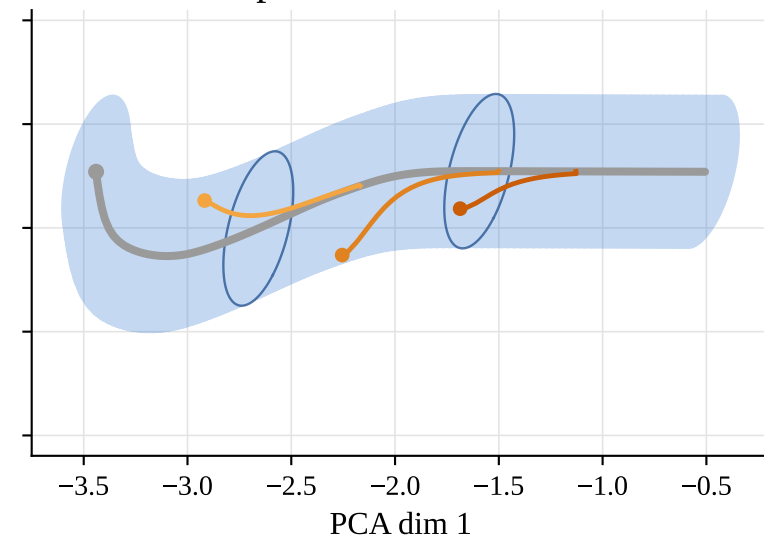
(d) Pooled \bar{\Sigma}^\alpha and sampled correction labels
