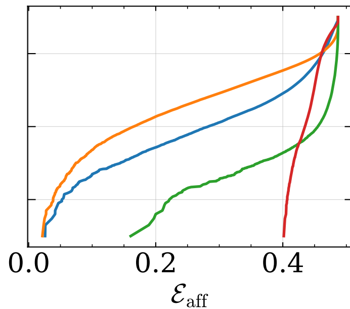
Sine
