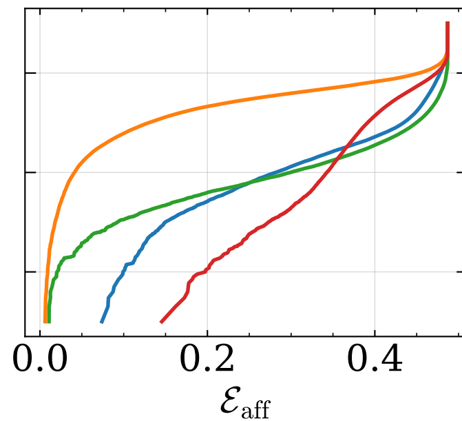
Parabola
