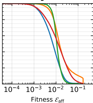
Sigmoid
