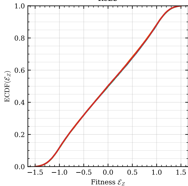
Parabola
