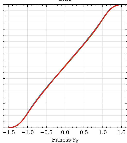
Sine
