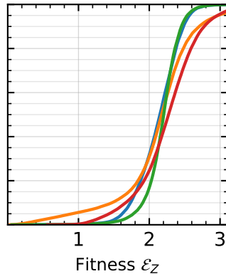
Parabola
