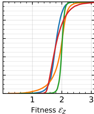
Sine
