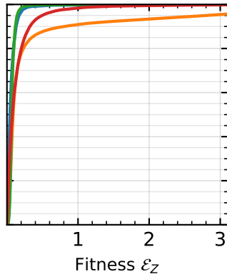
Sigmoid
