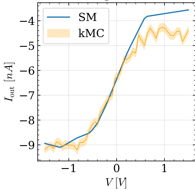
Sigmoid
