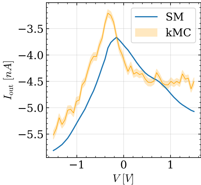
Cosine
